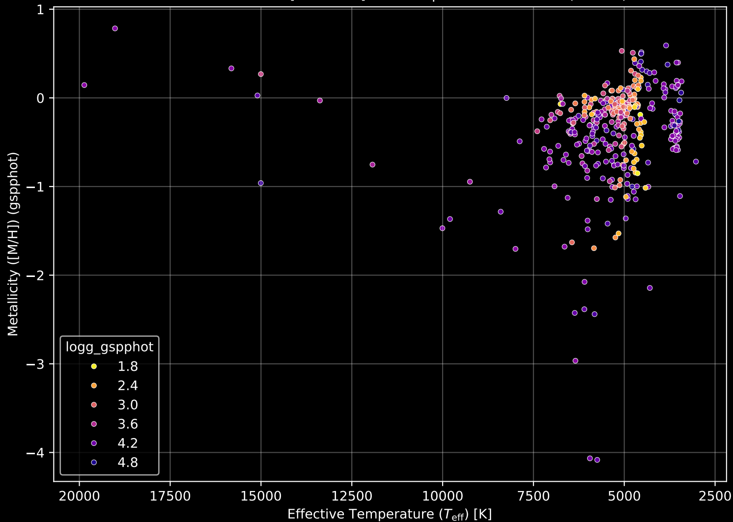
APOGEE DR17 Field: [ORIONB-B] Stellar Population Parameters (n= 384)
